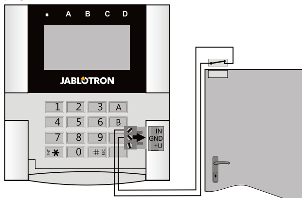
2. ábra: a nyitásérzékelő bekötése
