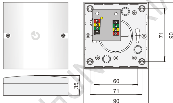
2. ábra: példa a modulnak a JA-190PL szerelődobozba történő telepítésére
