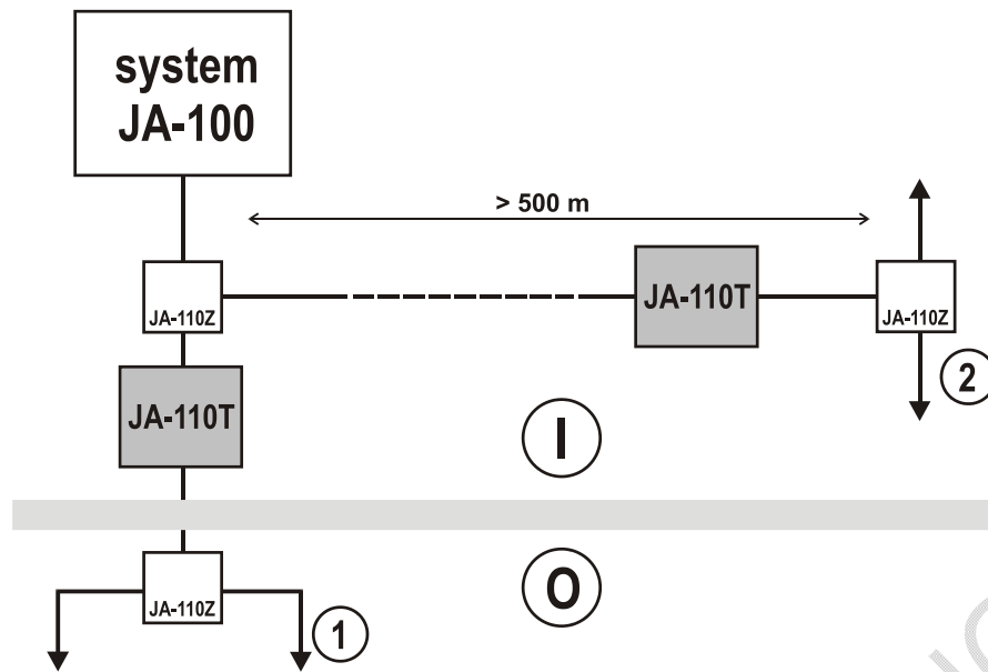
3. ábra: (I) belső (védett területen futó) vezetékszakasz; (O) külső (nem védett) területen futó adatbusz vezeték szakasz; (1) a külső vezetékszakasz leválasztása; (2) az adatbusz meghosszabbítása 500m-en felül (lásd - A leválasztó modul működése)
