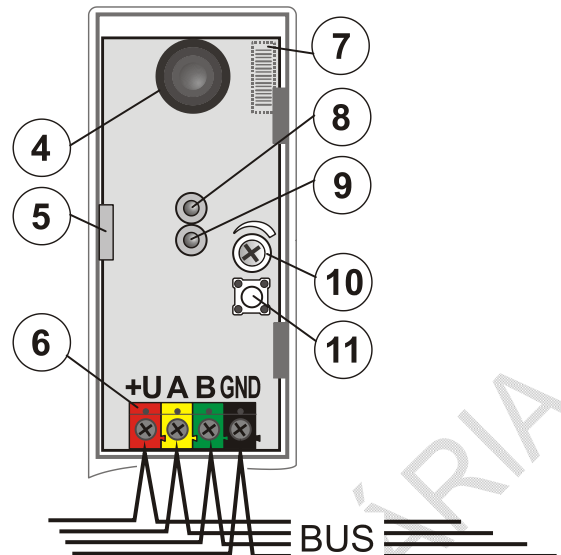
2. ábra: 4 – ŰT érzékelő; 5 – az áramköri lapot rögzítő műanyag nyelv; 6 – adatbusz sorcsatlakozója; 7 – vonalkód (a belső oldalon); 8 – az érzékelő aktiválását jelző piros visszajelző LED; 9 – sárga hibajelző LED; 10 – az érzékelő érzékenységének szabályozója; 11 – szabotázs kontaktus;
