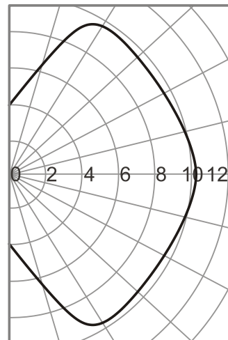
3. ábra: Az érzékelő érzékelési tartománya (felülnézet)
