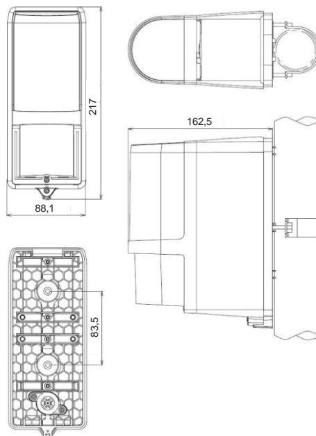
Fig. 9 Unit dimensions
